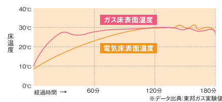
●立ち上がり特性(フローリング)
