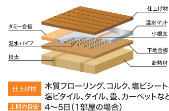
●「温水マット」構造図
