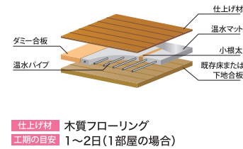
●「5.5mmマット」構造図
