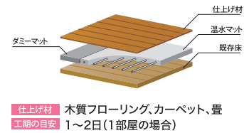
●「はやわざ」構造図
