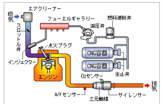
エルフCNG - MPI の燃料供給方式
